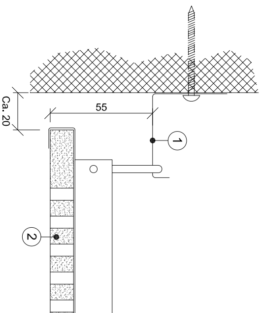
SNITT A-A
